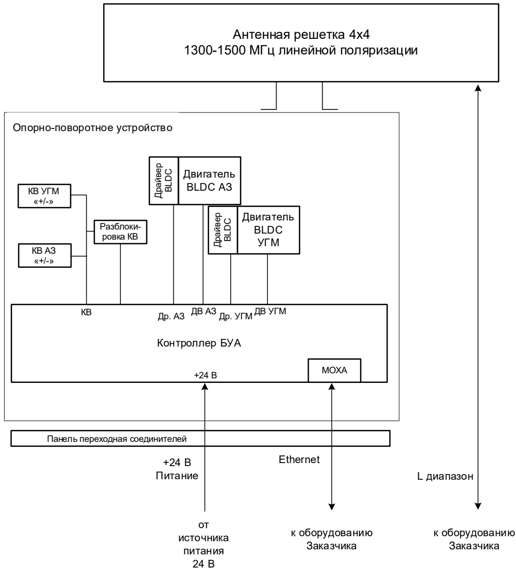
Рисунок 4 - Функциональная схема АС 4х4 L
