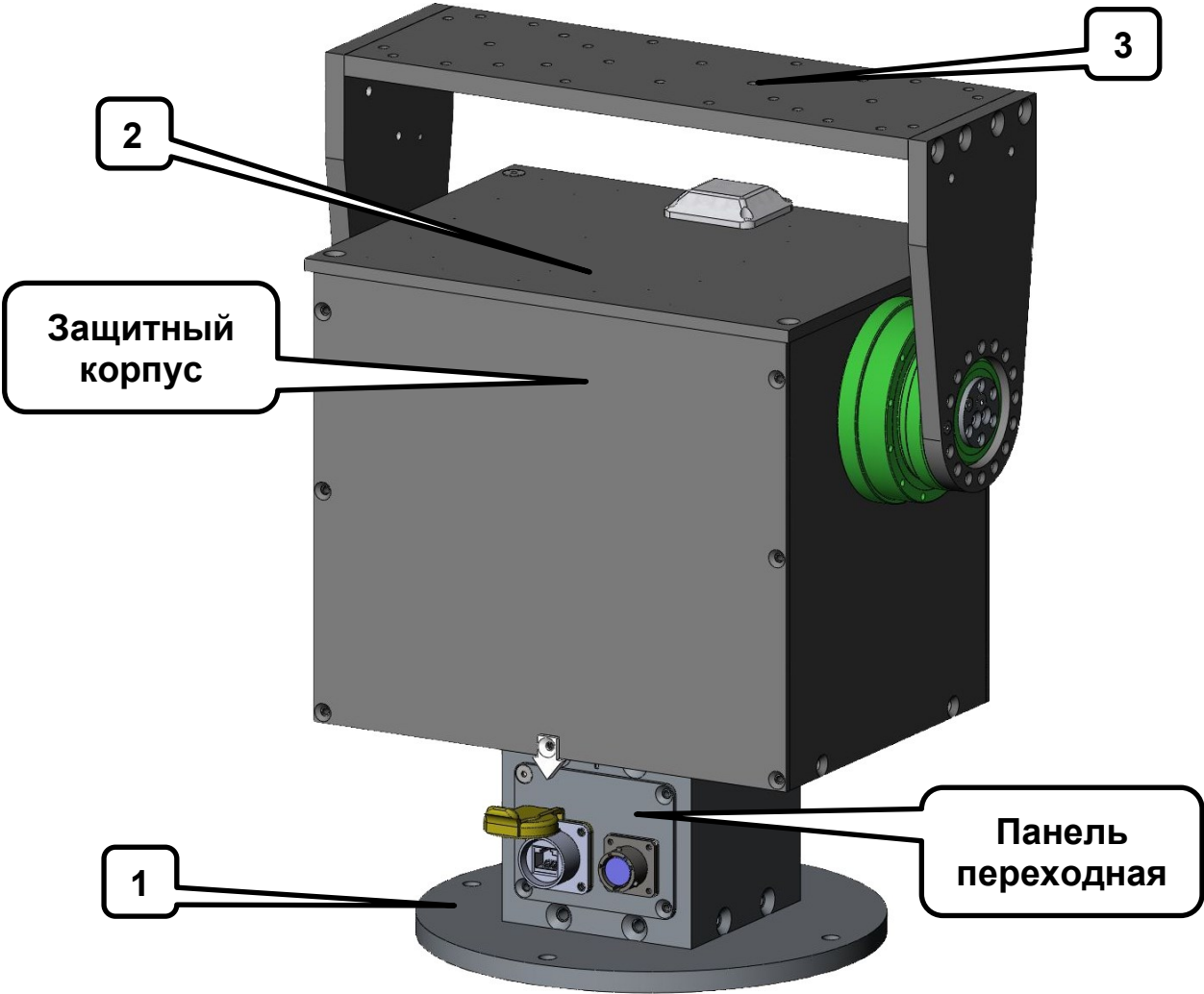
Рисунок 5 - Внешний вид ОПУ
