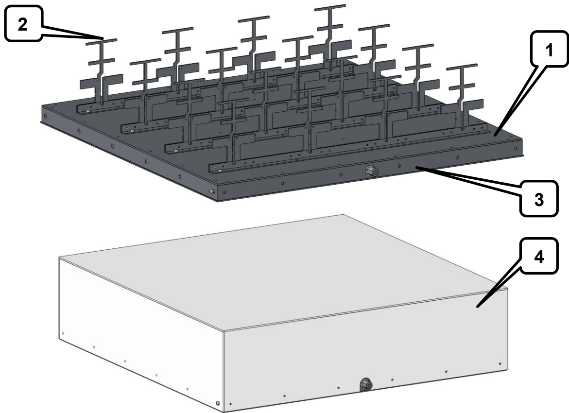
Рисунок 7 – Внешний вид антенной решетки 4х4 1300-1500 МГц линейной поляризации без РПУ и с РПУ
