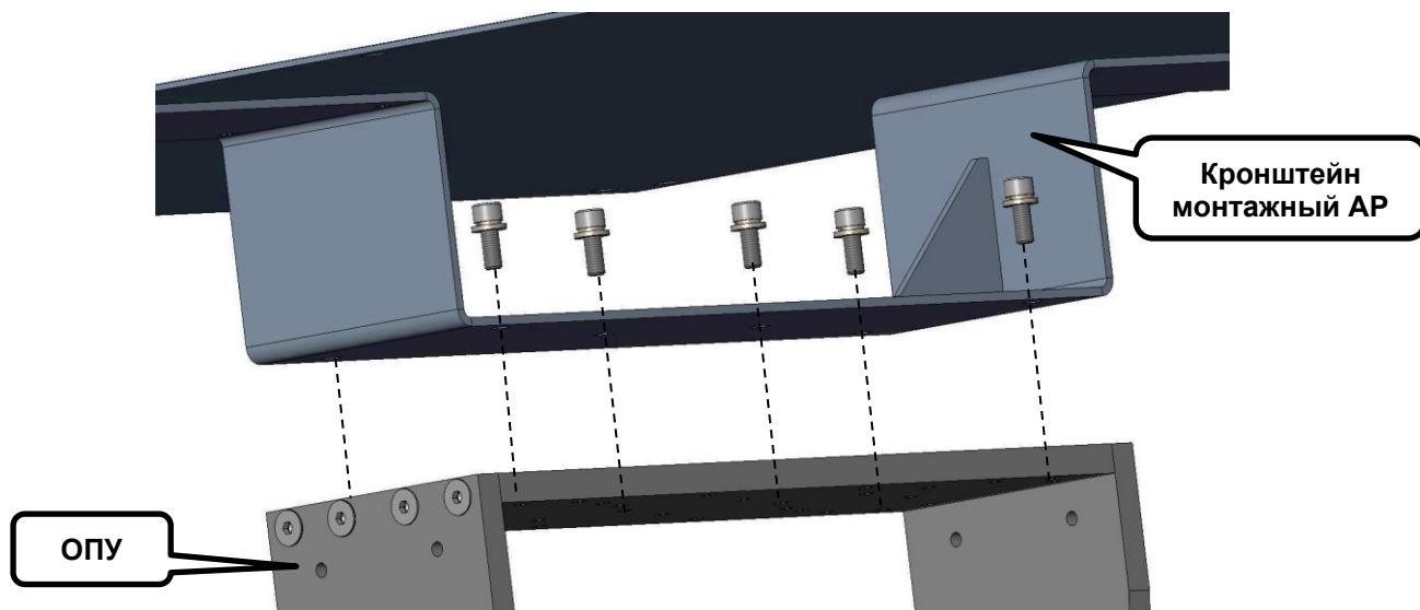
Рисунок 14 – Установка антенной решетки 4x4 на ОПУ
