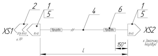
Рисунок 1 – монтаж разъема XS1 и XS2
