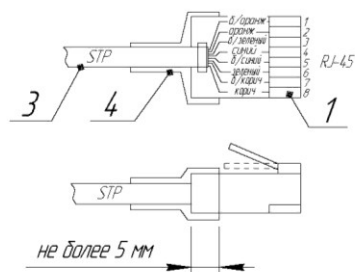
Рисунок 1 – монтаж разъема XS1 и XS2
