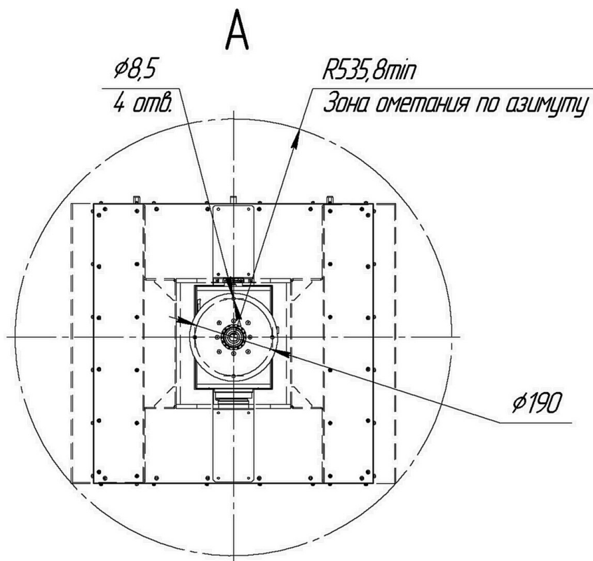
Рисунок 2 - Габаритный чертеж антенны в развернутом состоянии Внешний вид изделия представлены на рисунке 3.
