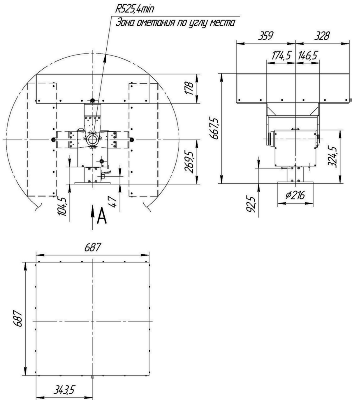
Рисунок 1 - Габаритный чертеж антенны в развернутом состоянии
