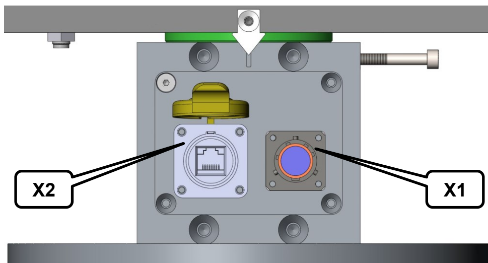
Рисунок 6 - Внешний вид переходной панели ОПУ.
