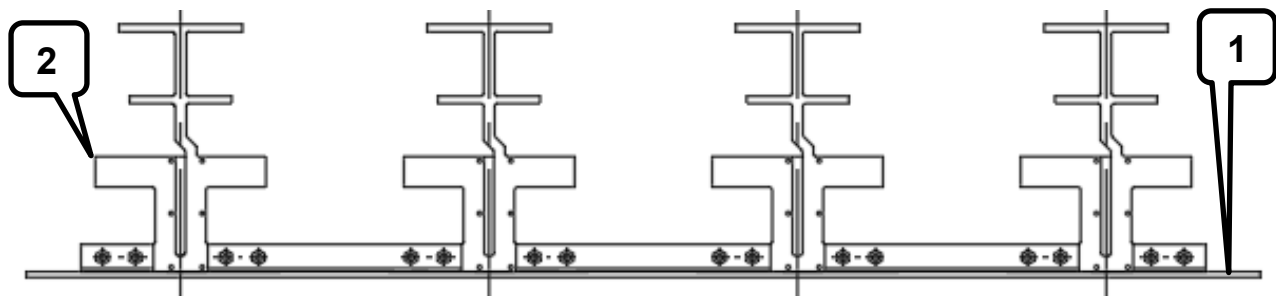
Рисунок 8 – Сечение антенной решетки и экрана
