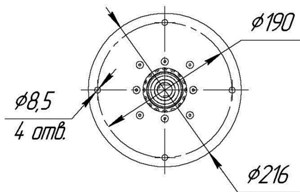
Рисунок 13 – Внешний вид установочного фланца ОПУ
